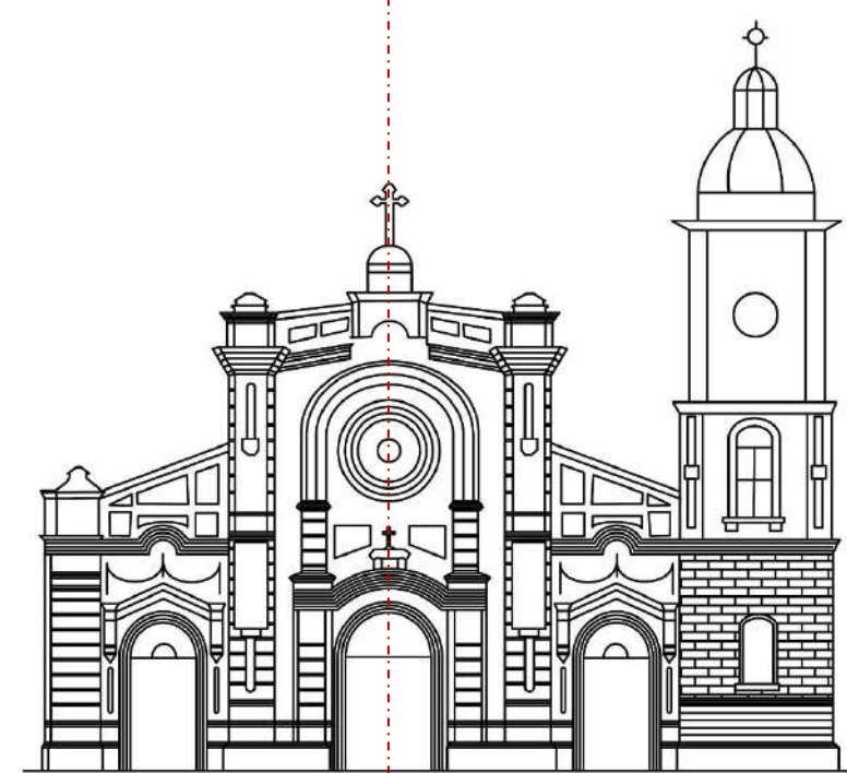
Levantamiento de la fachada principal / Main facade drawing . Fuente/ source: los autores / the authors
