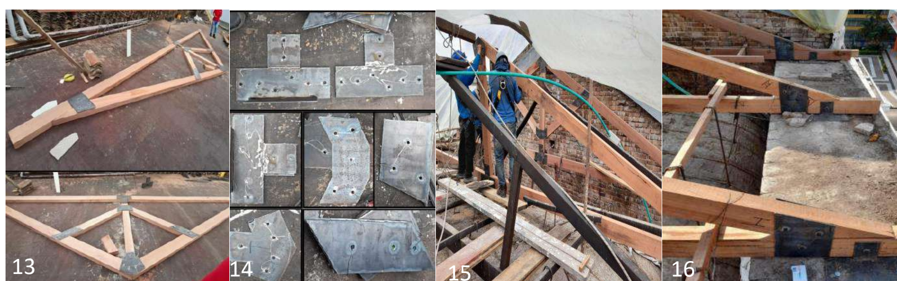
Imagen 13/16. montaje de las nuevas cerchas en la nave principal de la catedral / Assembly of the new trusses in the main nave of the Cathedral . Fuente/Source: Evangelista Nieto Devia
