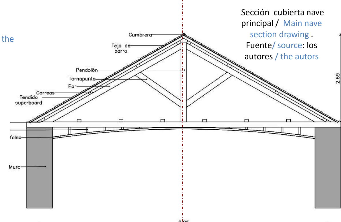
Sección transversal / Cross section/drawing . Fuente/ source: los autores / the autores
