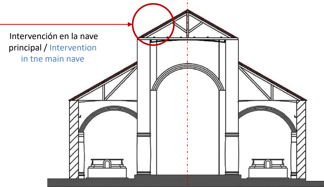
Sección transversal / Cross section/drawing . Fuente/ source: los autores / the autores
