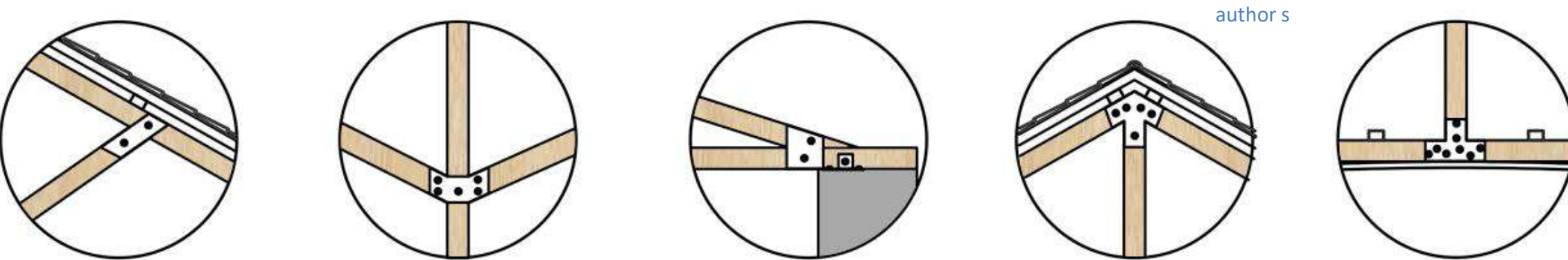
Detalles de unión de las cerchas de la nave principal / Details of the unions of the trusses of the main nave Fuente/ source: los autores/ the authors
