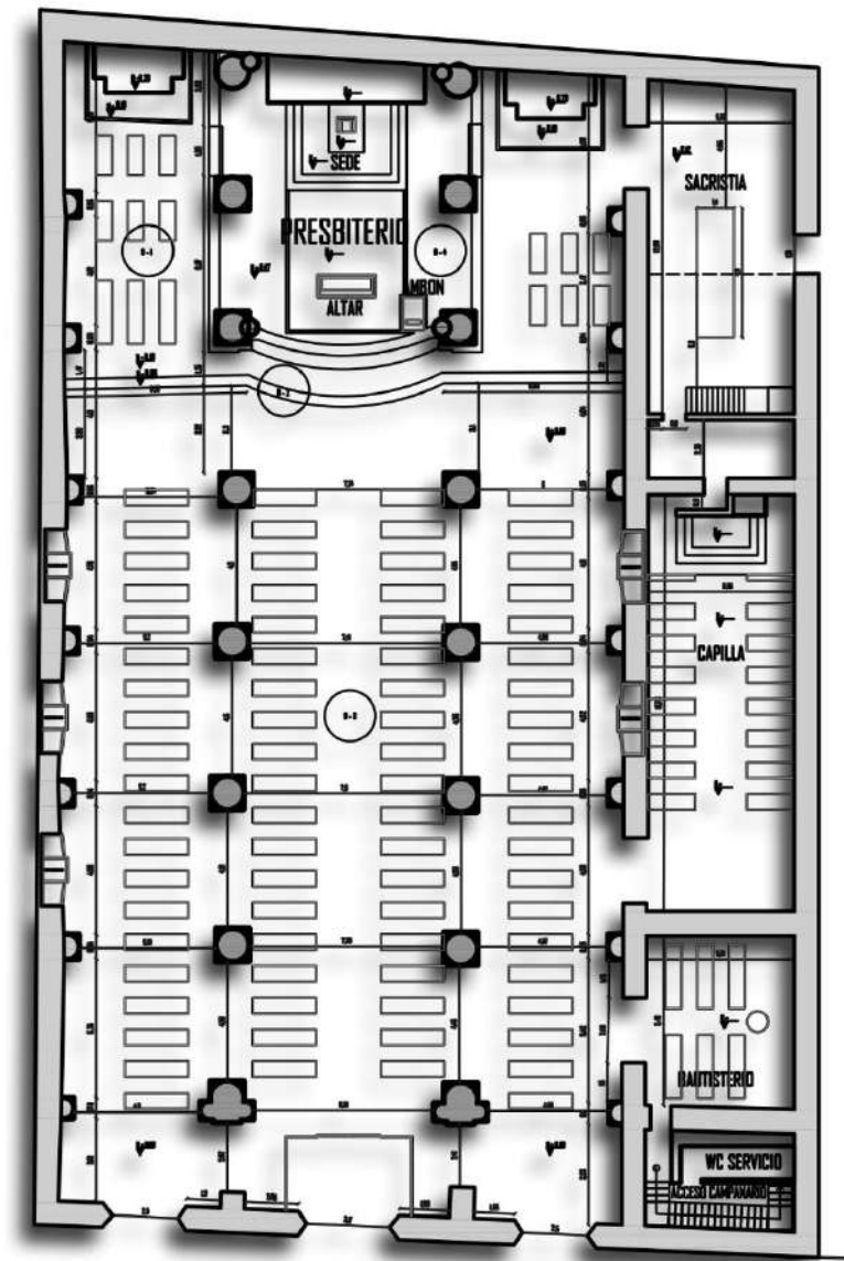
Levantamiento planta / Plan drawing . Fuente/ source: los autores/ the authors
